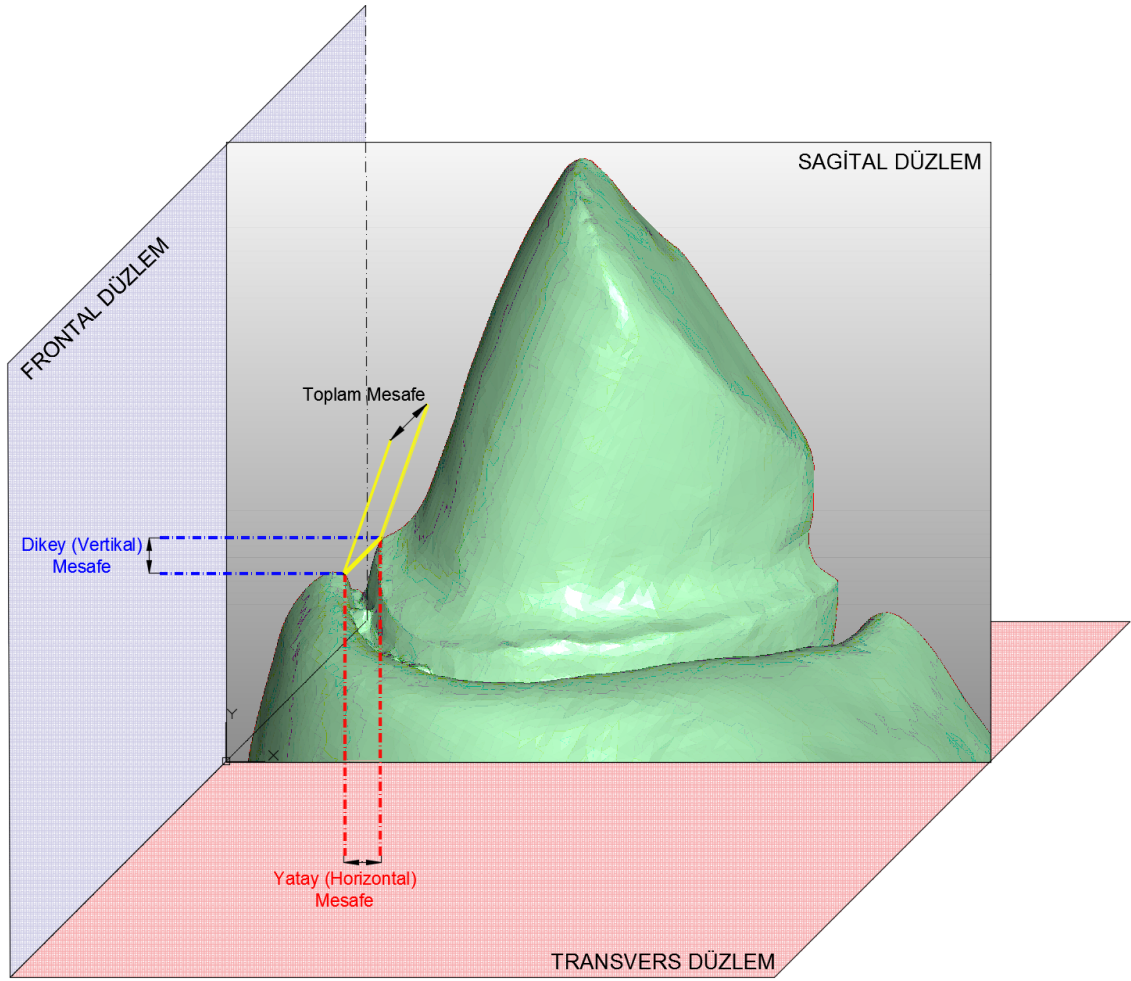
Şekil 3.18. Yatay, dikey ve toplam yer değiştirmenin düzlemler üzerinde gösterimi.
