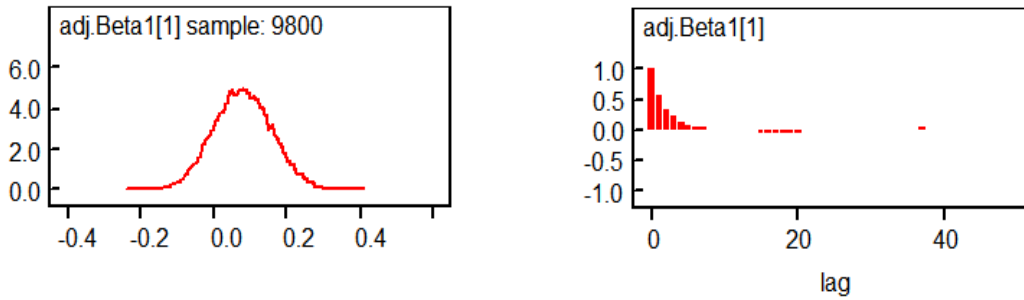
Birinci Madde için Yoğunluk (Density) ve Otokorelasyon (Autocorrelation) Grafikleri
