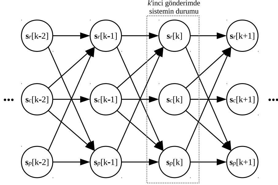
Şekil 4.2. C-NC-ARQ zamana bağlı durum modeli. Durum değişkenlerinin zamana bağlı değişen değerlerinin birbirleriyle olan ilişkisini göstermektedir.
