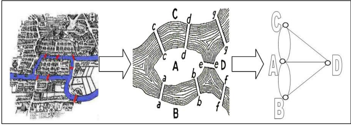
Şekil 1. Euler'in (1736) Königsberg kentinin köprülerini düğüm ve bağlar ile gösterimi.
