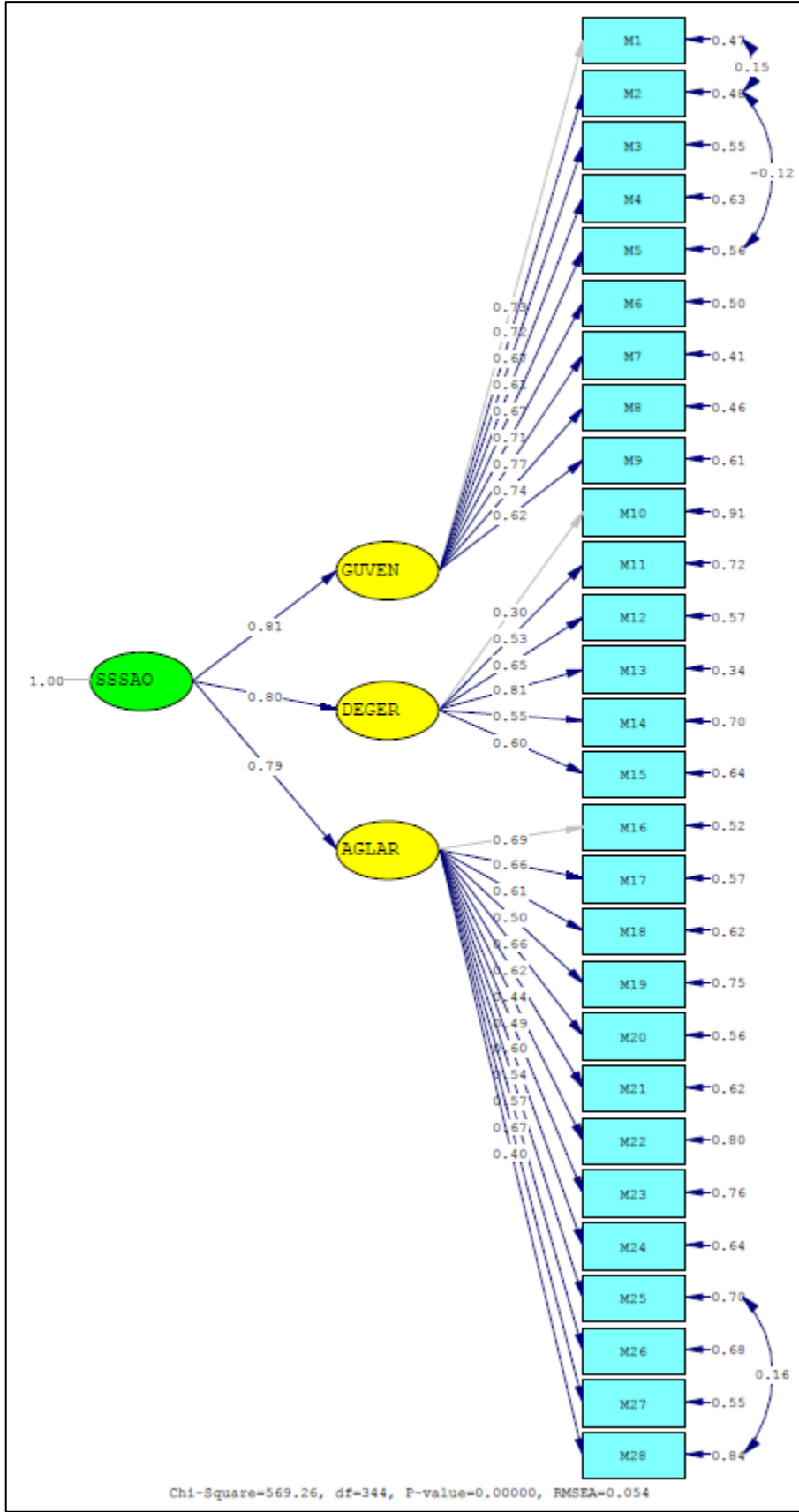
Şekil 9. Ölçeğe ait üç faktörlü path (yol) diyagramı.
