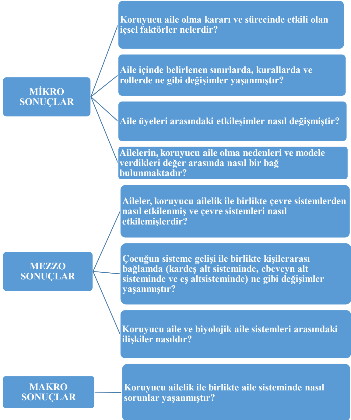
Şekil 16: Sonuçlar-Amaçlar Şeması
