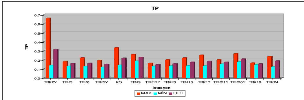
Şekil Ek 3.6. Toplam Fosfor Değişimleri
