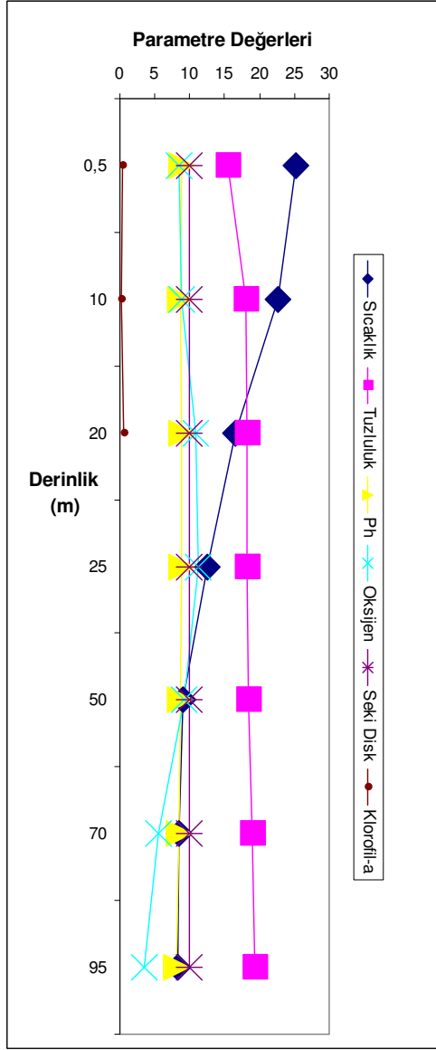
Şekil 3.17. İğneada (TRK3) İstasyonu Derinliğe Bağlı Fiziksel Parametre Değişimleri
