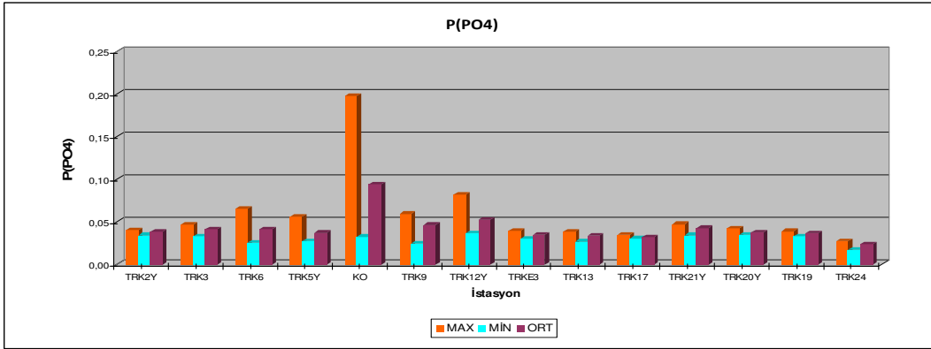
Şekil Ek 3.7. Fosfat Fosforu Deęişimleri
