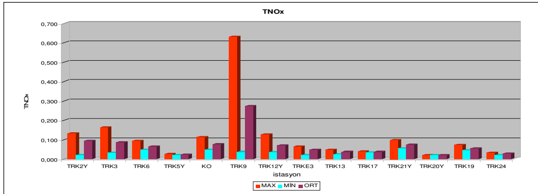
Şekil Ek 3.10. Toplam Oksitlenmiş Azot Değişimleri
