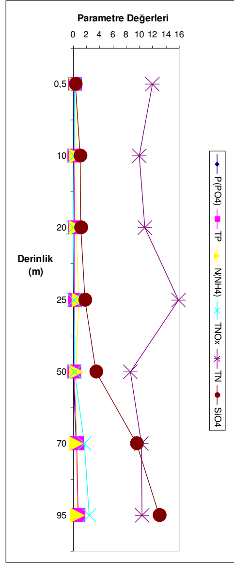
Şekil 3.18. İğneada (TRK3) İstasyonu Derinliğe Bağlı Besin Elementleri Değişimleri
