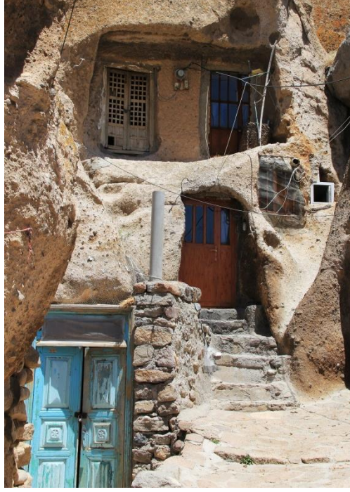
Şekil.3.14.kandovan evi kapılar. Kişisel arşiv
