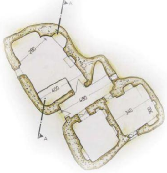
Şekil.3.17.kandovan dağ evi eskiz. Kişisel arşiv
