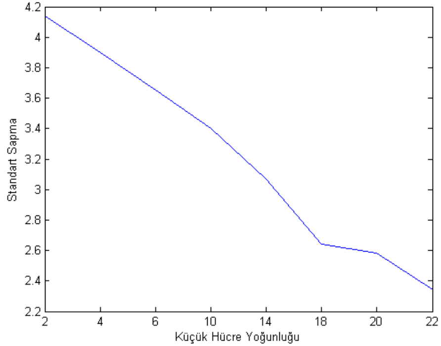
Şekil 5.11. Standart Sapma; V = 13,75 \text{ m/s} , d (hücre sayısı/ \text{km}^2 ) değişen küçük hücre yoğunluğu, gölgeleme sabiti 6, gönderilen güç değeri 200 mW ve T = 5 sn.
