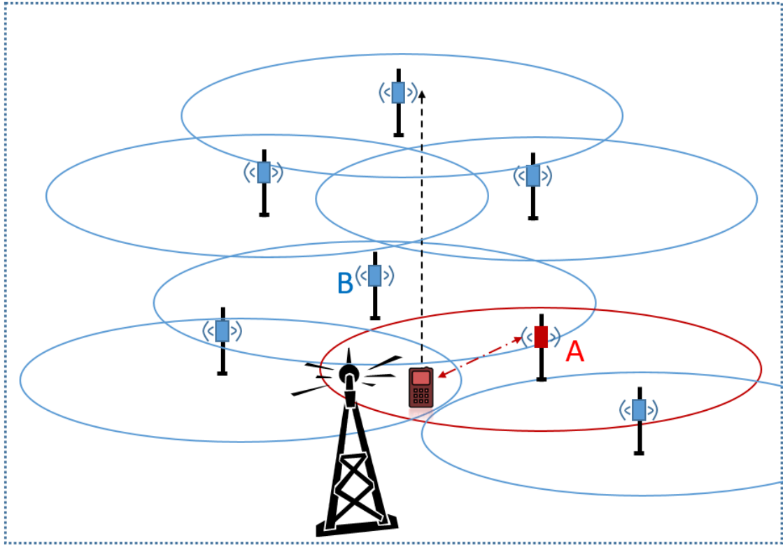
Şekil 2.6. t=0 anında mobil kullanıcı ve hücrelerin durumu
