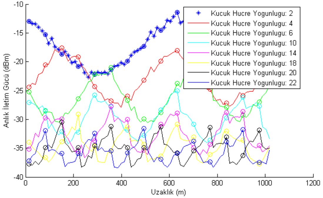
Şekil 5.16. Anlık İletilen Güç; V = 13,75 \text{ m/s} , d (hücre sayısı/ \text{km}^2 ) değişen küçük hücre yoğunluğu, gölgeleme sabiti 6, gönderilen güç değeri 200 mW ve T = 5 sn.
