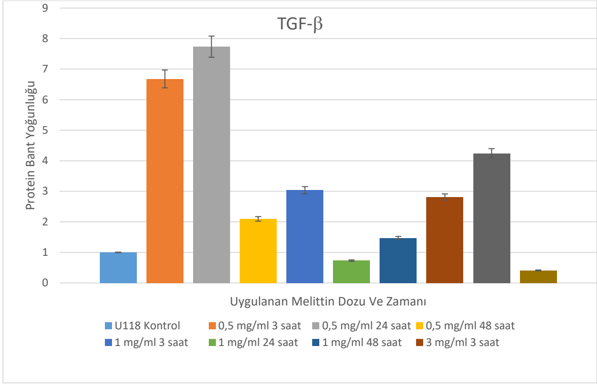
Şekil 4.12. TGF-β proteininin farklı doz ve zamandaki kat artışları grafiği
