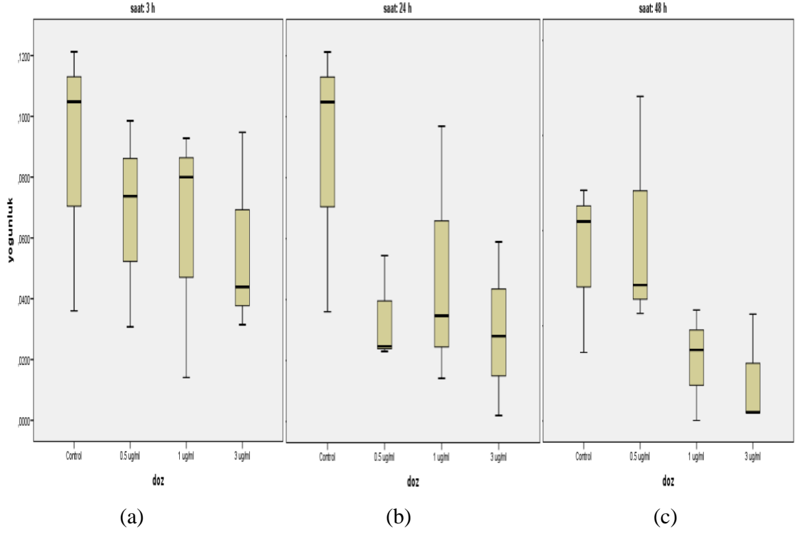
Şekil 4.16. ADAMTS-5 proteininin U118 kontrol hüresinin ve uygulanan 0,5, 1 ve 3 µg/ml konsantrasyondaki Melittin dozunun 3 saatlik (a), 24 saatlik (b), 48 saatlik (c) uygulama box-plot grafiği
