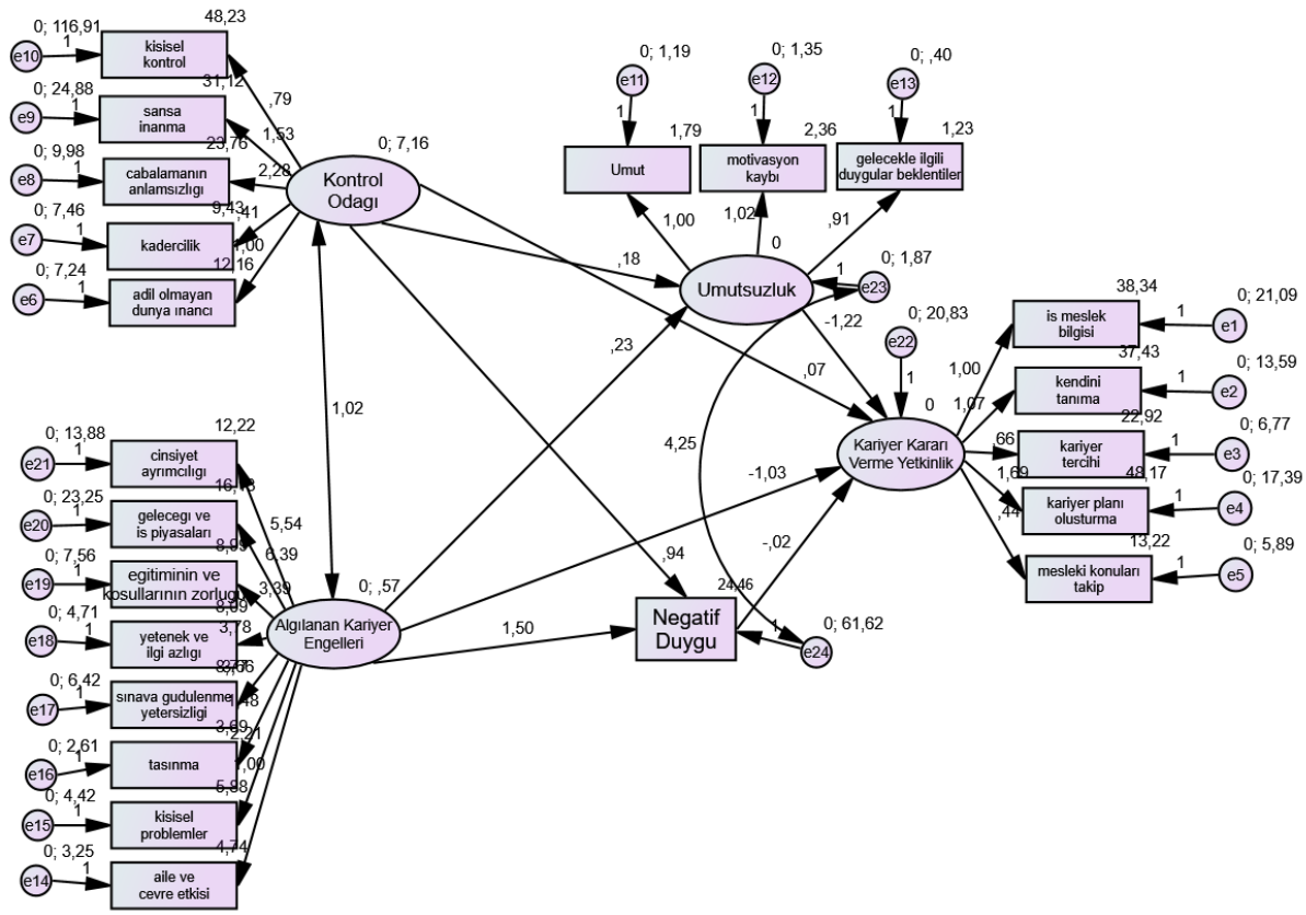
Şekil 4.5. Yapısal Model
