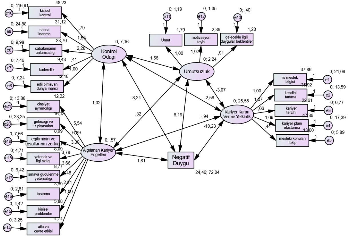
Şekil 4.4. Ölçüm Modeli
