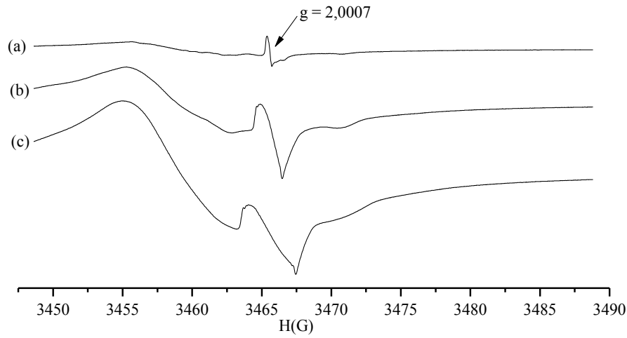
Őekil 4.8. Yapay iřınlama dozu 2291 Gy olan IC3-B-8 rneėinin (a) 0,4 G, (b) 2 G (c) 4 G modlasyon genliėi kullanılarak kaydedilen ESR spektrumları.
