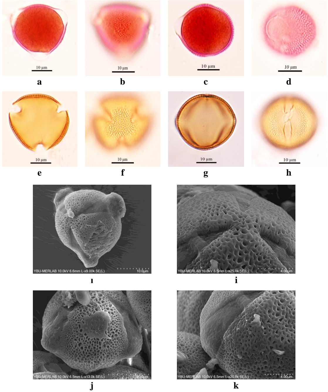
Şekil 4.9. V. vulcanicum var. vulcanicum 'un polen mikrofotografaları (a-h: LM, i-k: SEM)
