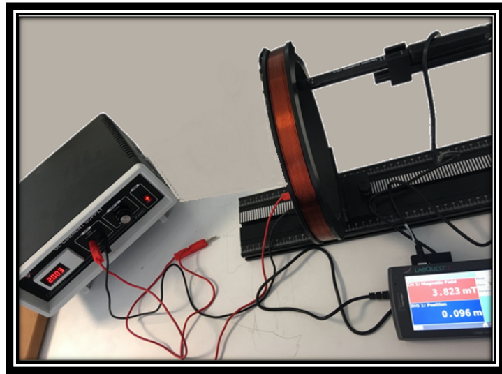
Şekil 18. y-ekseninde bobinin iç kısmında merkezden farklı bir noktada (üst tellere yakın) oluşan manyetik alan durumu ( I:2.0 A, B:3.82 mT, r_x:0.09 m).
