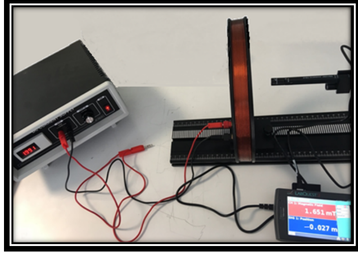
Şekil 23. Bobine pozitif yönde akım uygulandığında oluşan manyetik alan durumu ( I:2.0 A, B:1.65 mT, r_x:-0.02 m).
