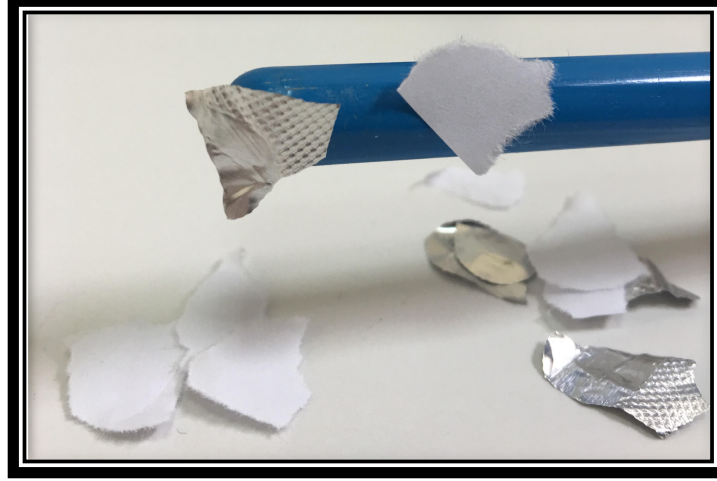
Şekil 10. Daha kuvvetli bir elektrik alanın yakınındaki nötr iletken folyolara ve nötr yalıtkan kağıtlara etkisi.
