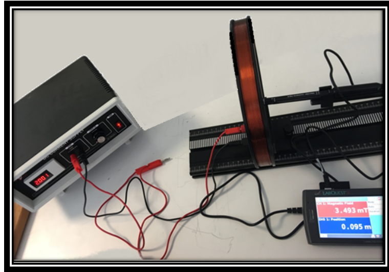
Şekil 20. y-ekseninde bobinin iç kısmında merkezden farklı bir noktada (alt tellere yakın) oluşan manyetik alan durumu ( I:2.0\text{ A} , B:3.49\text{ mT} , r_x:0.09\text{ m} ).
