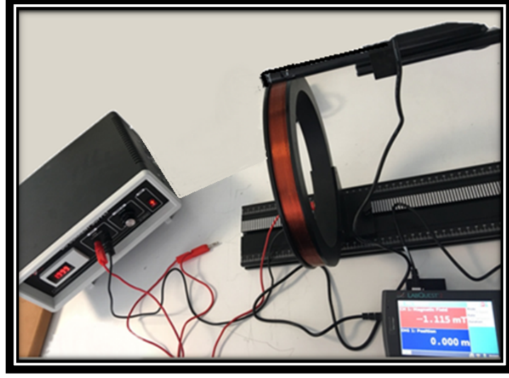
Şekil 21. y-ekseninde bobinin dış kısmında tellere yakın bir noktada oluşan manyetik alan durumu (I:2.0 A, B:-1.11 mT).
