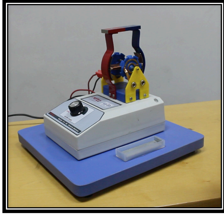
Şekil 38. Dış manyetik alandaki akım ilmeğinin tork sıfır olduğundaki durumu.
