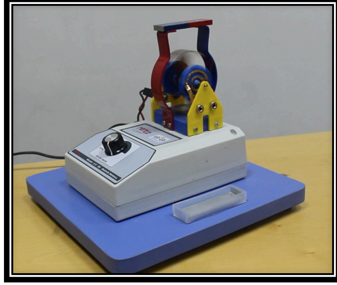
Şekil 41. Dış manyetik kuvvetin yönünün 180 derece değiştirildiği durum.
