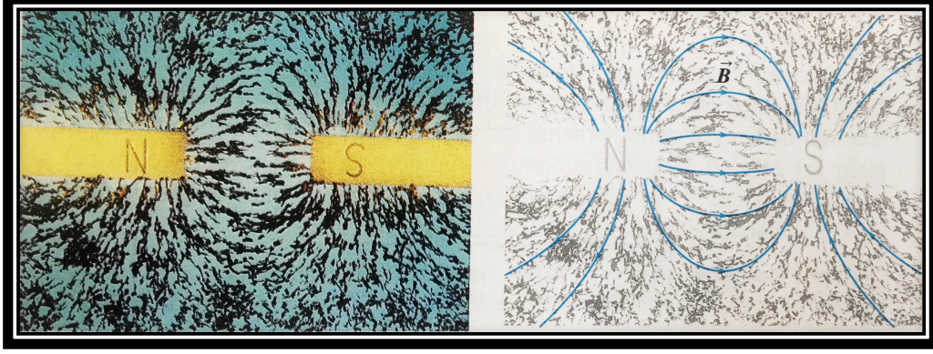
Şekil 71. İki ayrı mıknatısın oluşturduğu manyetik alan örneği 1 (Young & Freedman, 2010).
