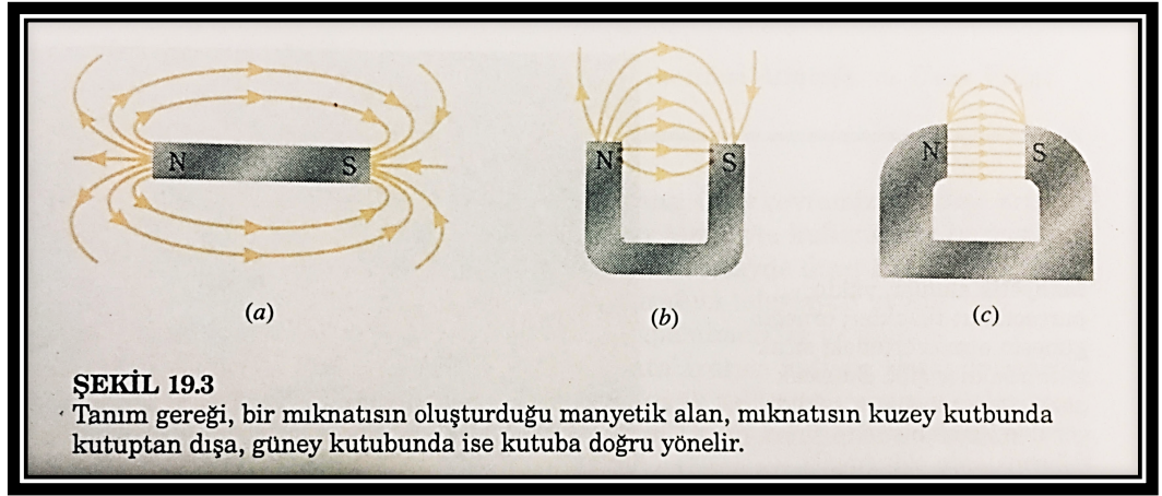
Şekil 74. Mıknatısın oluşturduğu manyetik alan örneği 1 (Bueche & Jerde, 2010).
