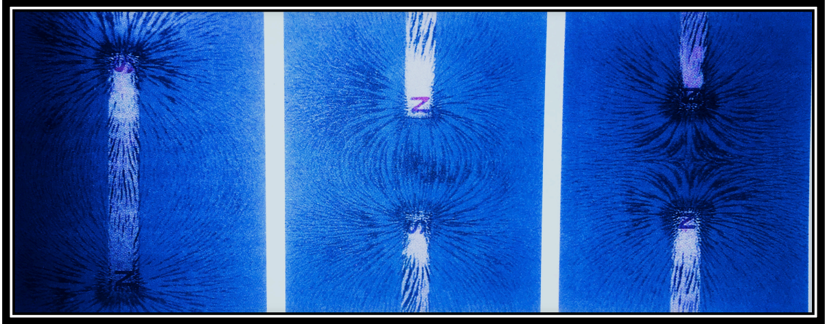
Şekil 72. İki ayrı mıknatısın oluşturduğu manyetik alan örneği 2 (Serway & Beicher, 2007).
