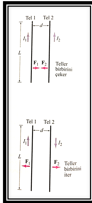
Şekil 79. Manyetik kuvvet konusunun anlatılması (Fishbane vd., 2003).
