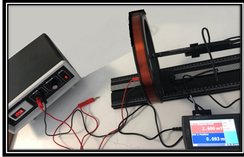
Şekil 19. y-ekseninde bobinin merkezinde oluşan manyetik alan durumu ( I:2.0\text{ A} , B:2.60\text{ mT} , r_x:0.09\text{ m} ).
