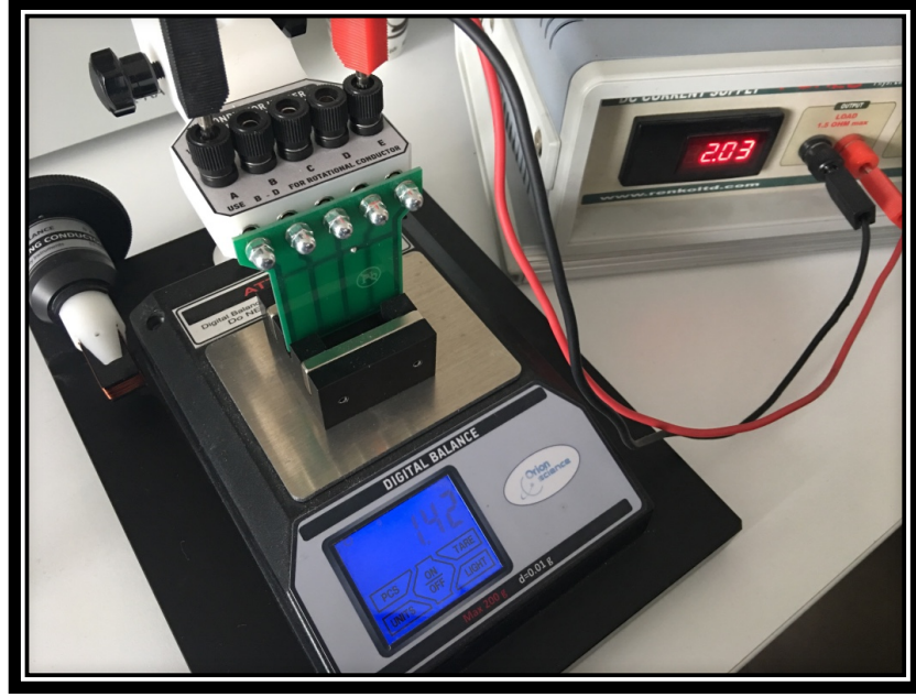
Şekil 32. Akım geçen tele sayfa düzleminden dışarı doğru etkiyen manyetik alanın büyüklüğü (küçük manyetik alan, tartıda okunan değer:1.42, manyetik alan yönü:
