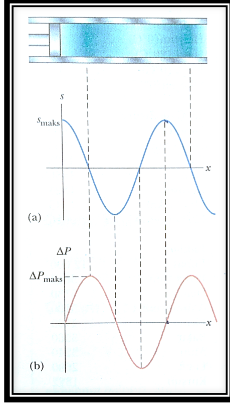
Şekil 67. Sinüzoidal ses dalgasının yerdeğiştirme-konum ve basın-konum grafiği örneği 1 (Serway & Beicher, 2002).
