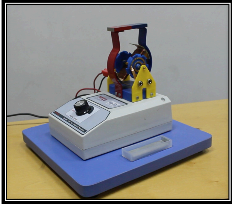
Şekil 39. Dış manyetik alandaki akım ilmeğinin tork sıfırdan farklı olduğundaki durumu.
