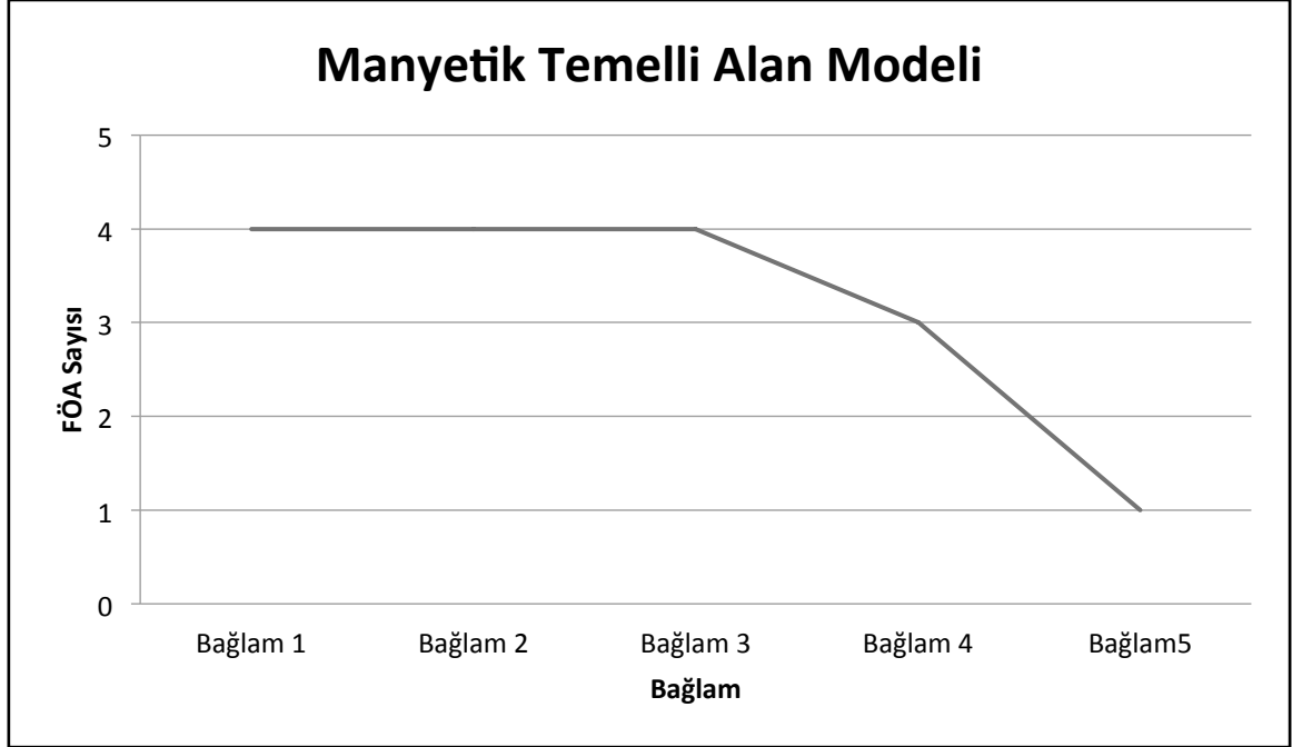
Şekil 43. Manyetik Temelli Alan Modeli-Bağlam ilişkisi.
