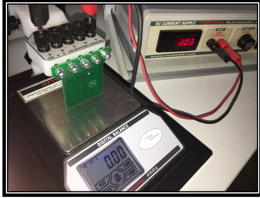
Şekil 37. Akım geçen tele dış manyetik alan uygulanmadığında manyetik kuvvet durumu ( I > 0 , tartıda okunan değer: 0.0, B: 0.0).
