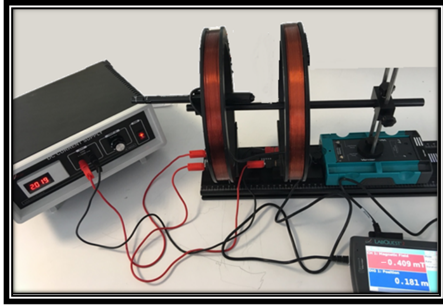
Şekil 28. Bobinlerden zıt yönlü akım aktığında ikinci bobinin dışında oluşan manyetik alan durumu ( I:2.0 A, B:-0.40 mT, r_x:0.18 m).
