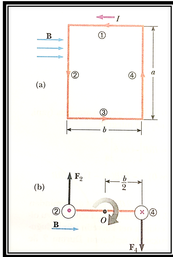
Şekil 78. Akım halkasının dış manyetik alanda bulunma durumu örneği 1 (Serway & Beicher, 2007).
