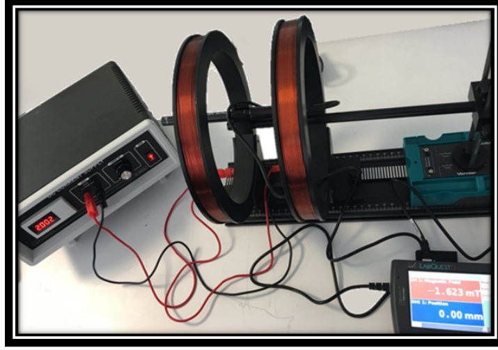
Şekil 31. Bobinlerden aynı yönlü akım aktığında ikinci bobinin dışında oluşan manyetik alan durumu ( I:2.0 A, B:-1.62 mT, r_x:0.0 m).
