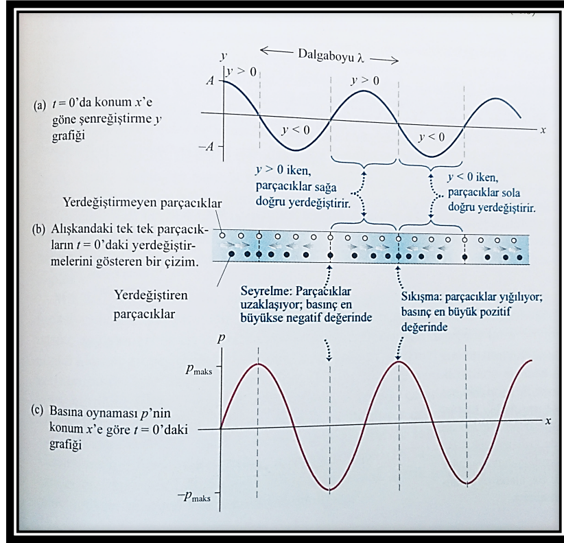
Şekil 68. Sinüzoidal ses dalgasının yerdeğiştirme-konum ve basın-konum grafiği örneği 2 (Young & Freedman, 2009).
