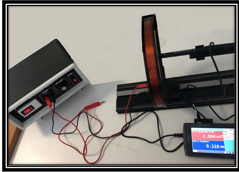
Şekil 16. x-ekseninde bobinin merkezinde oluşan manyetik alan ( I:2.0\text{ A} , B:2.50\text{ mT} , r_x:0.11\text{ m} ).
