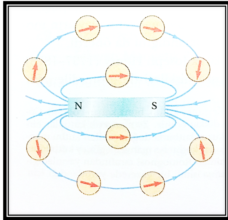
Şekil 75. Mıknatısın oluşturduğu manyetik alan örneği 2 (Serway & Beicher, 2007).
