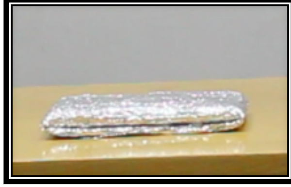
Şekil 12. Elektrik alanın kapalı iletken yüzeydeki durumu.
