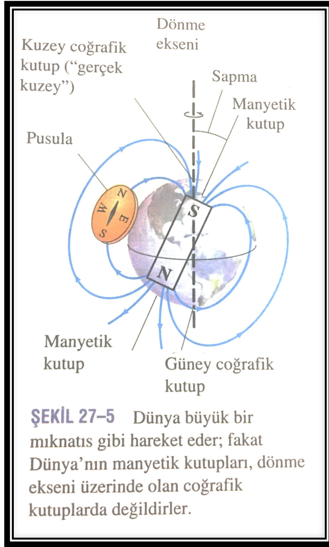
Şekil 76. Dünya'nın oluşturduğu manyetik alan (Giancoli, 2009).
