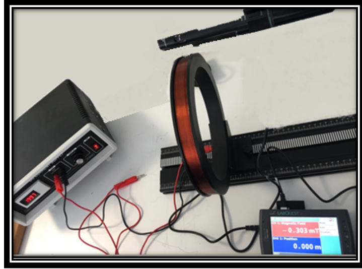
Şekil 22. y-ekseninde bobinin dış kısmında tellere uzak bir noktada oluşan manyetik alan durumu (I:2.0 A, B:-0.30 mT).
