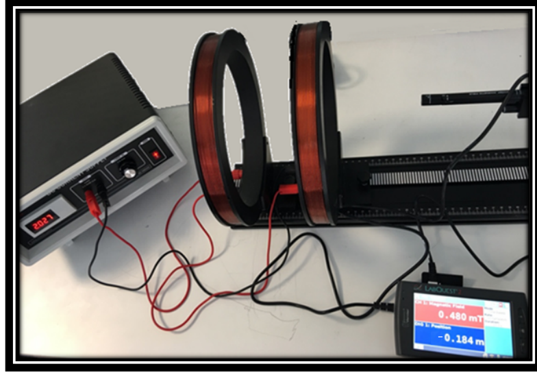
Şekil 26. Bobinlerden zıt yönlü akım aktığında birinci bobinin dışında oluşan manyetik alan durumu ( I:2.0 A, B:0.48 mT, r_x:-0.18 m).
