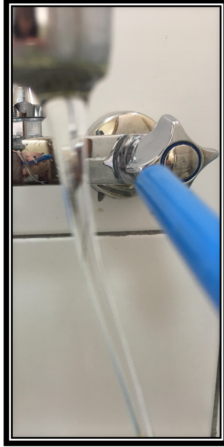
Şekil 11. Elektrik alanın nötr iletken suya etkisi.
