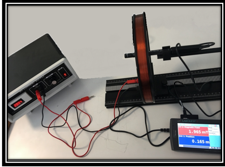
Şekil 17. x-ekseninde bobinin merkezinden uzaklaşırken herhangi bir noktada oluşan manyetik alan durumu ( I:2.0 A, B:1.96 mT, r_x:0.16 m).
