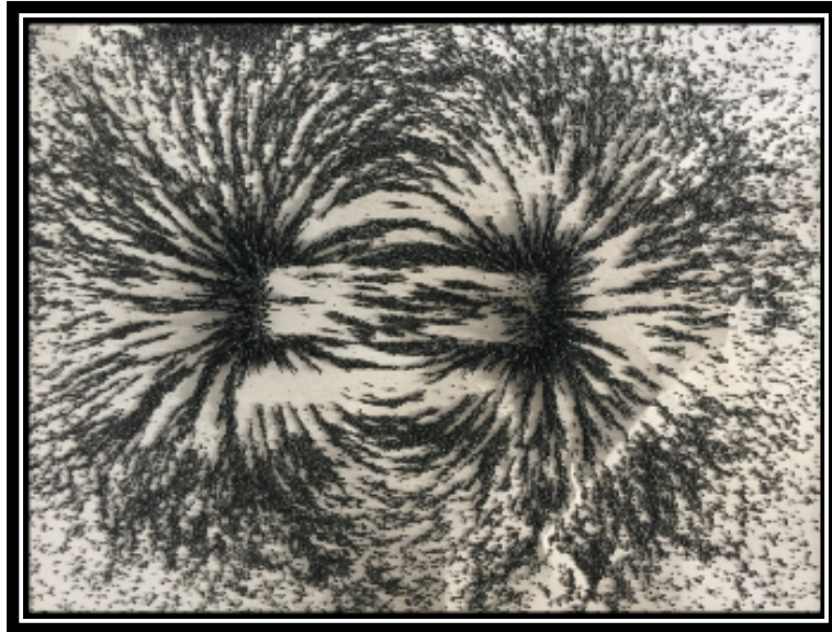
Şekil 14. Demir tozları yardımıyla mıknatısın manyetik alanının gösterimi.
