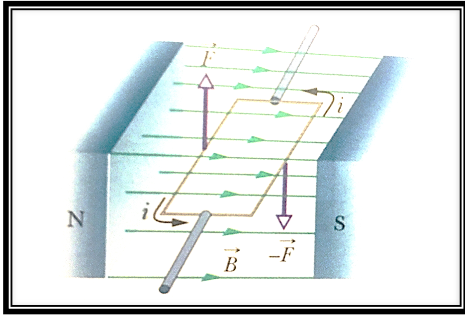
Şekil 77. Akım halkasının dış manyetik alanda bulunma durumu örneği 1 (Halliday vd., 2014).
