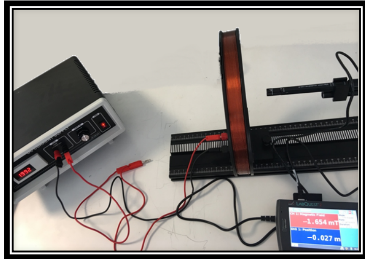
Şekil 24. Bobine negatif yönde akım uygulandığında oluşan manyetik alan durumu ( I:-2.0 A, B:-1.65 mT, r_x:-0.02 m).
