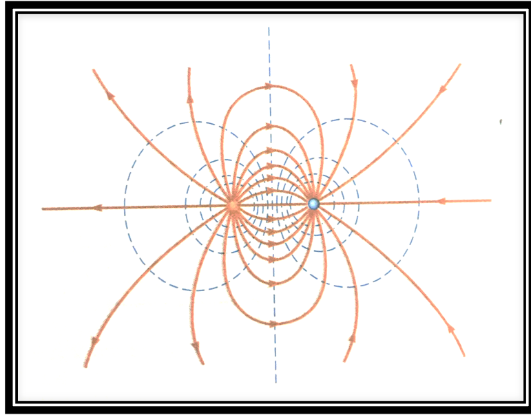
Şekil 66. Eşpotansiyel yüzey örneği 2 (Serway & Beicher, 2007).
