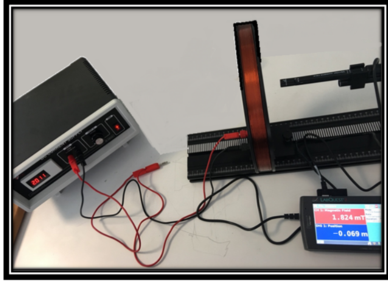
Şekil 15. x-ekseninde bobinin merkezine yaklaşıırken herhangi bir noktada oluşan manyetik alan durumu ( I:2.0\text{ A} , B:1.82\text{ mT} , r_x:-0.06\text{ m} ).
