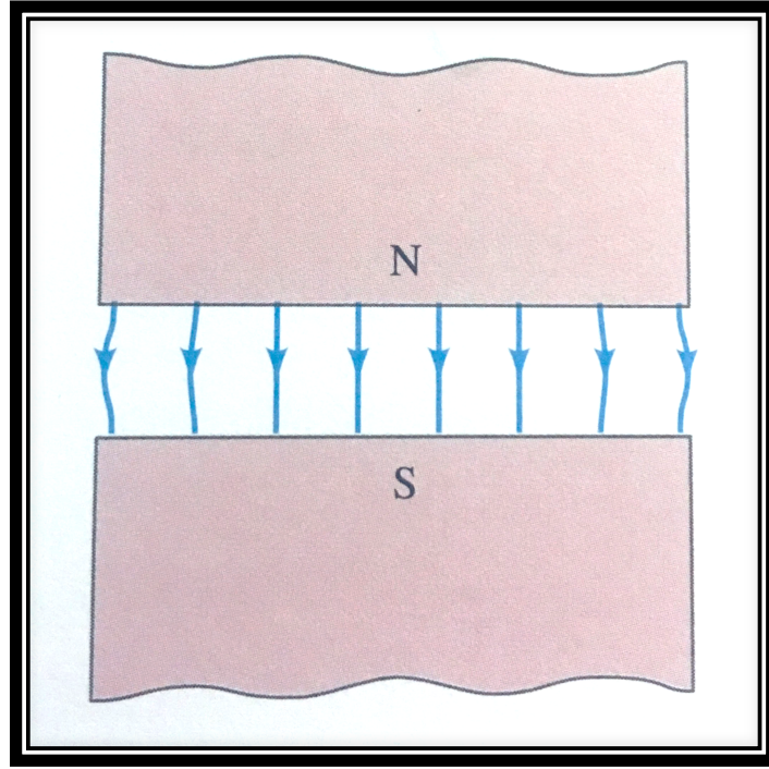
Şekil 73. İki ayrı mıknatısın oluşturduğu manyetik alan örneği 3 (Giancoli, 2009).
