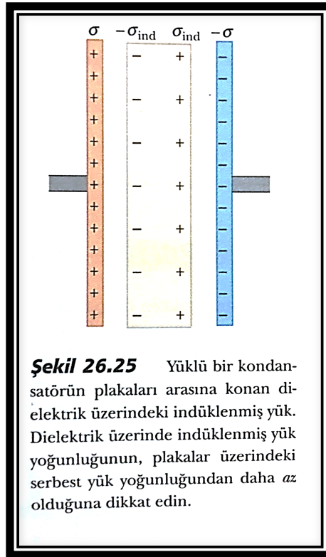
Şekil 64. Yüklü bir kondansatör örneği (Serway & Beicher, 2007).
