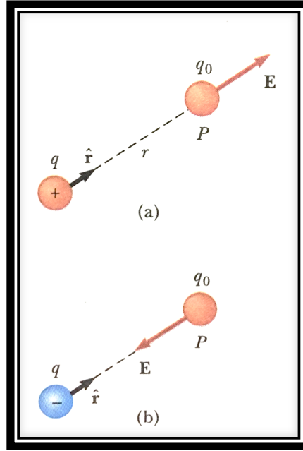
Şekil 63. Yük-deneme yükü ilişkisi (Serway & Beicher, 2007).
