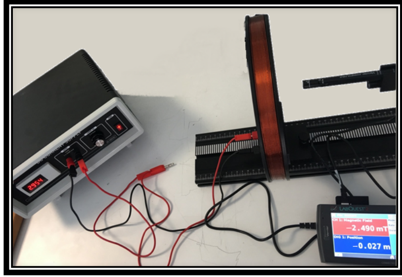
Şekil 25. Bobine pozitif yönde akım uygulandığında oluşan manyetik alanın büyüklüğünün artırıldığı durum ( I:3.0\text{ A} , B:-2.49\text{ mT} , r_x:-0.02\text{ m} ).
