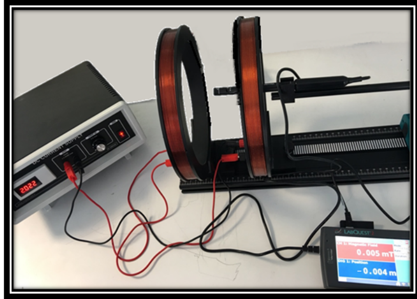
Şekil 27. Bobinlerden zıt yönlü akım aktığında iç bölgenin orta noktasında oluşan manyetik alan durumu ( I:2.0 A, B:0.00 mT, r_x:-0.0 m).
