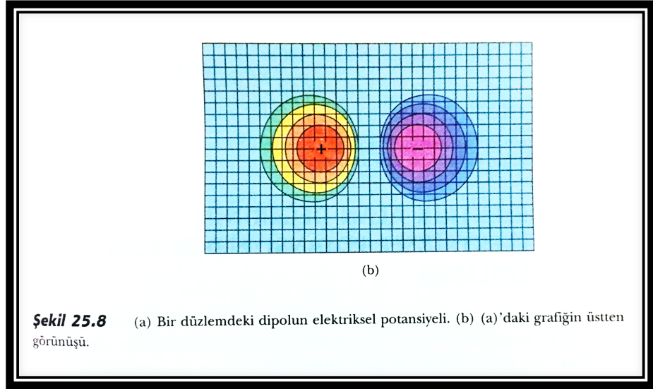
Şekil 65. Eşpotansiyel yüzey örneği 1 (Serway & Beicher, 2007)
