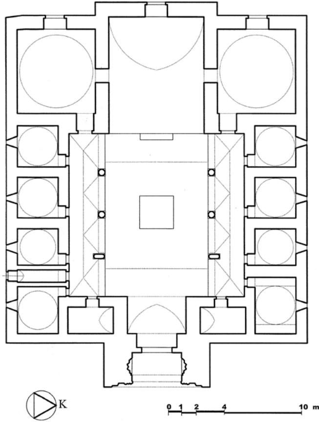
Çizim 16. Karaman Hatuniye Medresesi Planı, (O. N. Dülgerler, 2006).
