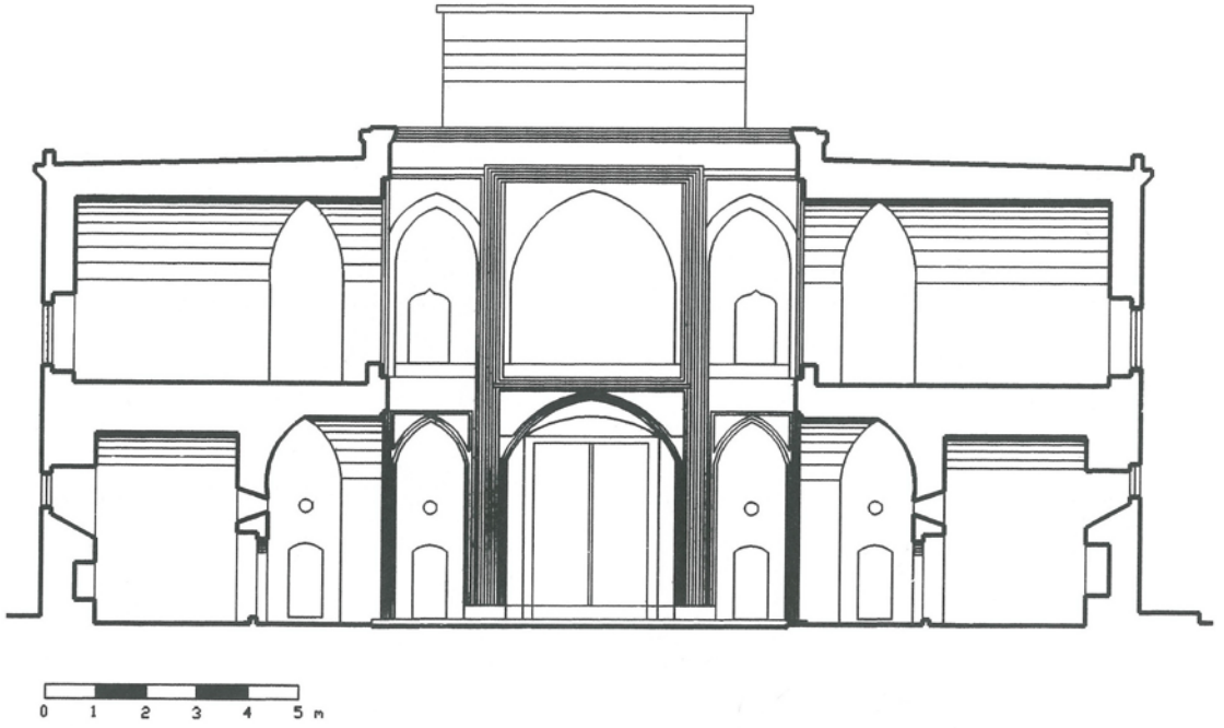
Çizim 10. Medrese, C-C kesiti (M. Özkarcı, 2001).
