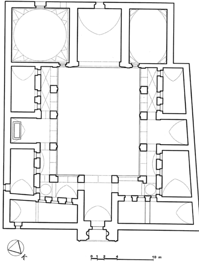
Çizim 12. Aksaray Zincirli Medresesi Planı, (A. Kuran, 1969).
