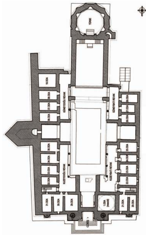
Çizim 19: Erzurum Çifte Minareli Medrese Üst Kat Planı (M. Sezer, 2015).
