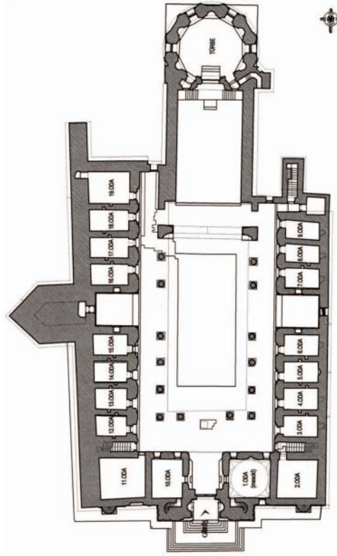
Çizim 18. Erzurum Çifte Minareli Medrese Zemin Kat Planı (M. Sezer, 2015).
