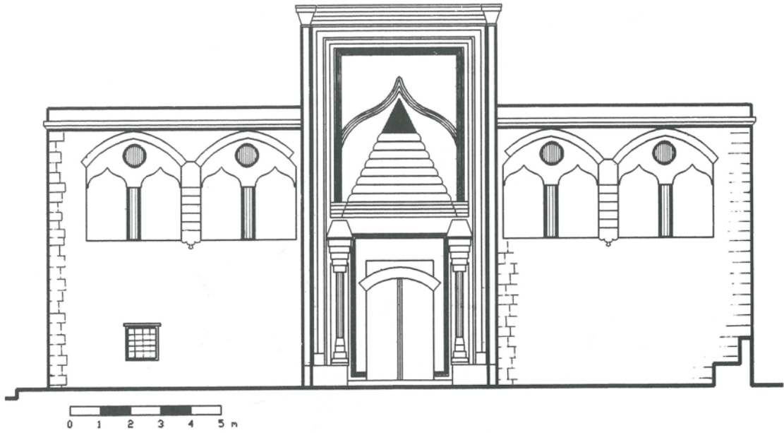
Çizim 7. Kuzey/ön cephe, (M. Özkarcı, 2001).
