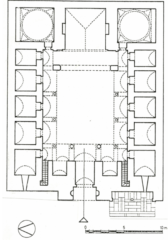
Çizim 24. Kayseri Hatuniye Medresesi Planı (M. Sözen, 1970).
