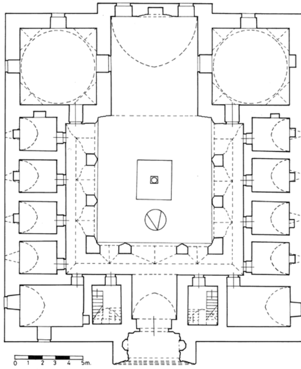
Çizim 2. Niğde Ak Medrese Alt Kat Planı (M. Özkarcı, 2001).
