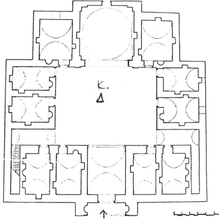
Çizim 23. Beçin Ahmet Gazi Medresesi Planı (A. Arel, 1968).
