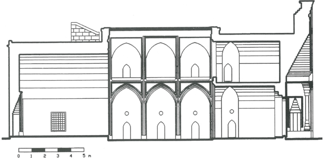
Çizim 8. Medrese, A-A kesiti (M. Özkarcı, 2001).
