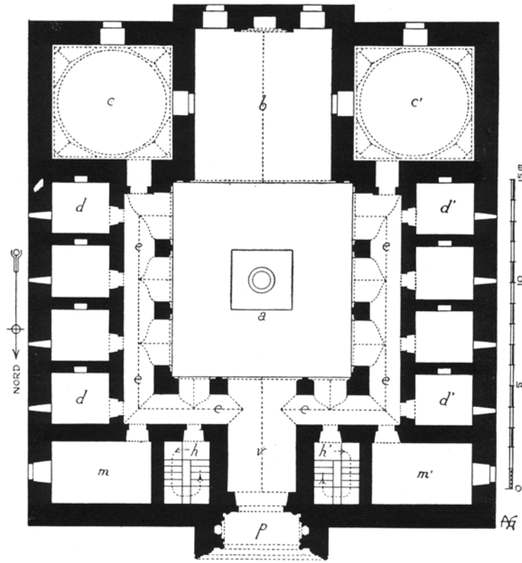
Çizim 4. Niğde Ak Medrese Alt Kat Planı (A. Gabriel, 1931).
