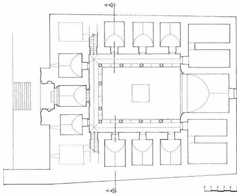
Çizim 20. Eğirdir Dündar Bey Medresesi Planı (VGM Arşivinden).
