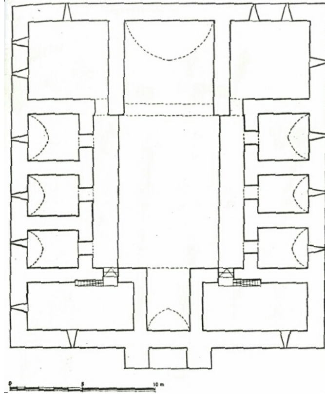
Çizim 22. Korkuteli Emir Sinaneddin Medresesi Üst Kat Planı (M. Sözen, 1970).
