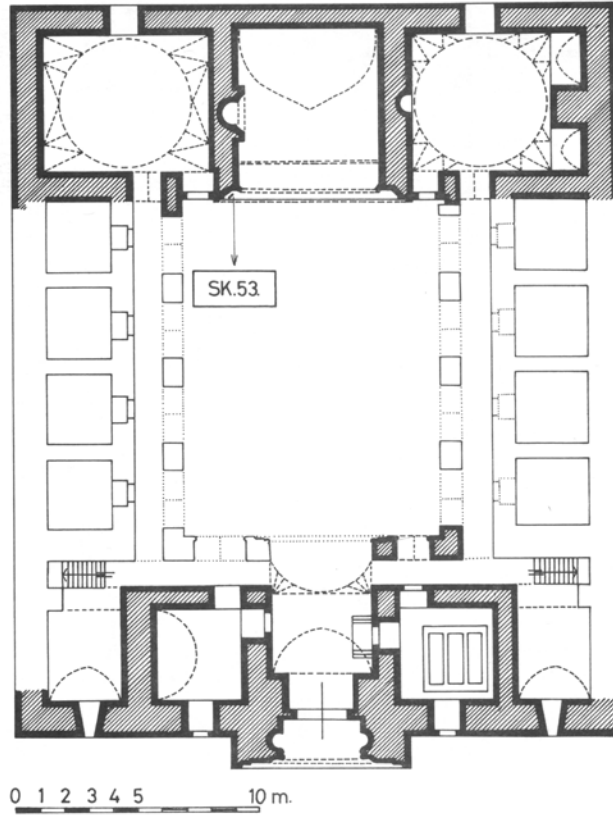
Çizim 17. Konya Sırçalı/Bedreddin Muslih Medresesi Planı (Z. Sönmez, 1995).
