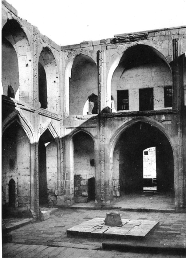
Fotoğraf 5. Niğde Ak Medrese, ayrıntı, (A. Gabriel, 1931).
