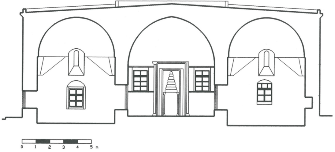
Çizim 9. Medrese, B-B kesiti (M. Özkarcı, 2001).
