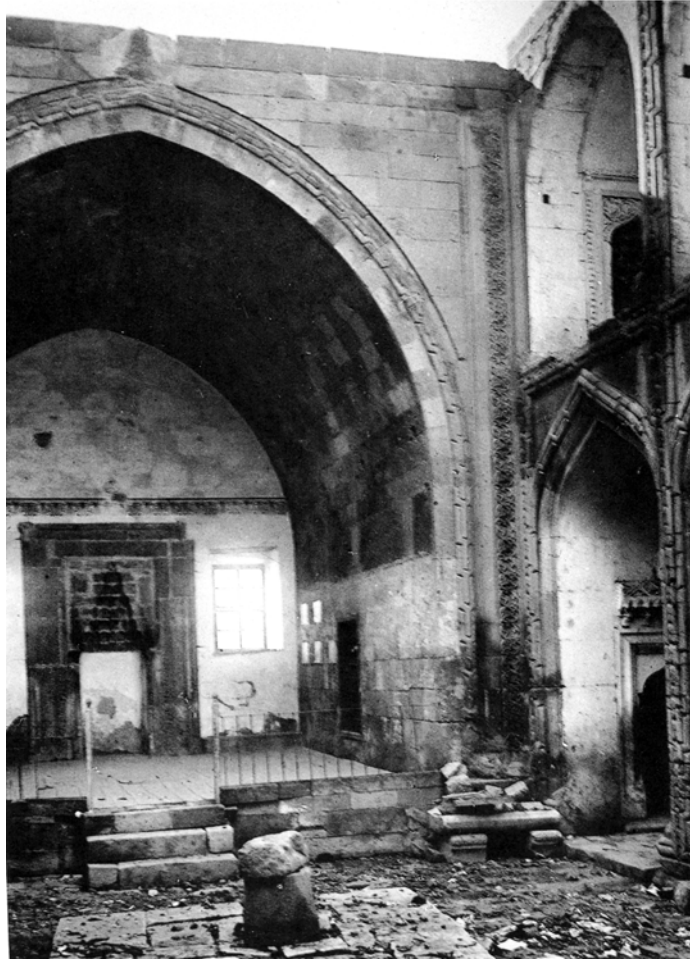
Fotoğraf 7. Niğde Ak Medrese, eyvan, ayrıntı, (A. Gabriel, 1931).
