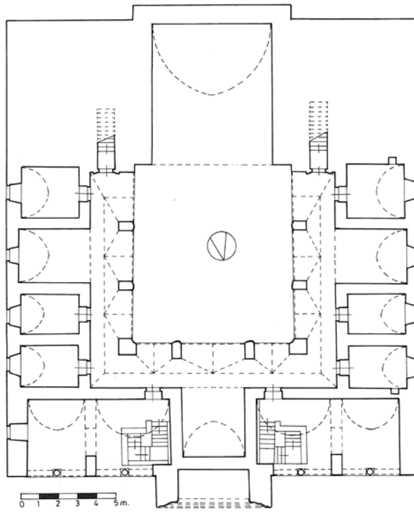
Çizim 3. Niğde Ak Medrese Üst Kat Planı (M. Özkarcı, 2001).
