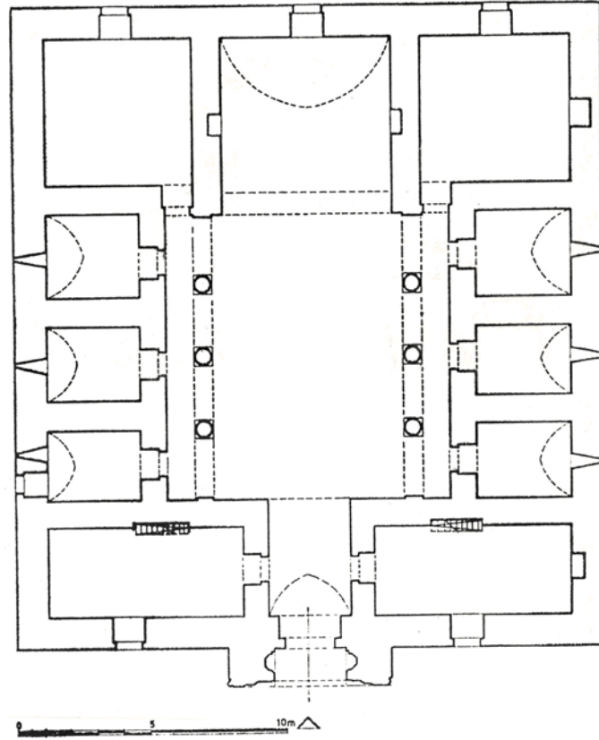
Çizim 21. Korkuteli Emir Sinaneddin Medresesi Zemin Kat Planı (M. Sözen, 1970).
