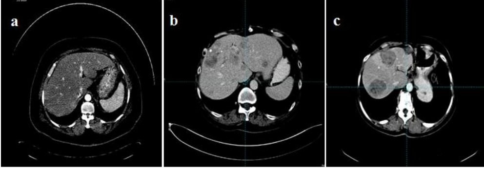
Şekil 4.96. 5mm kesit kalınlığında elde edilmiş a) B.60 b) B.30 c) B.20 konvolüsyon filtreli BT görüntüleri
