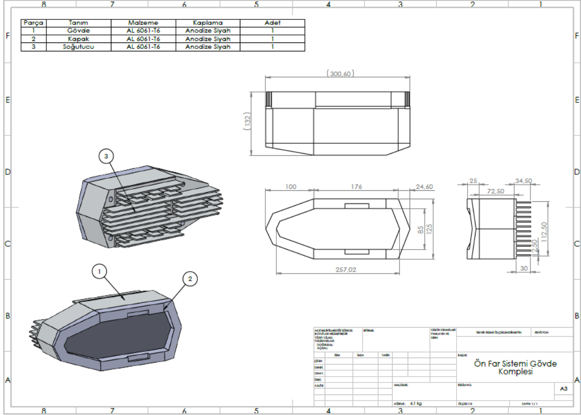
Ek-1: Ön Far Sistemi Gövde Kompleksi Teknik Resmi
