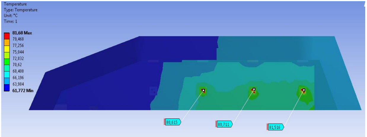
Şekil 12-7 Uzun hüzme modu analiz sonuçları
