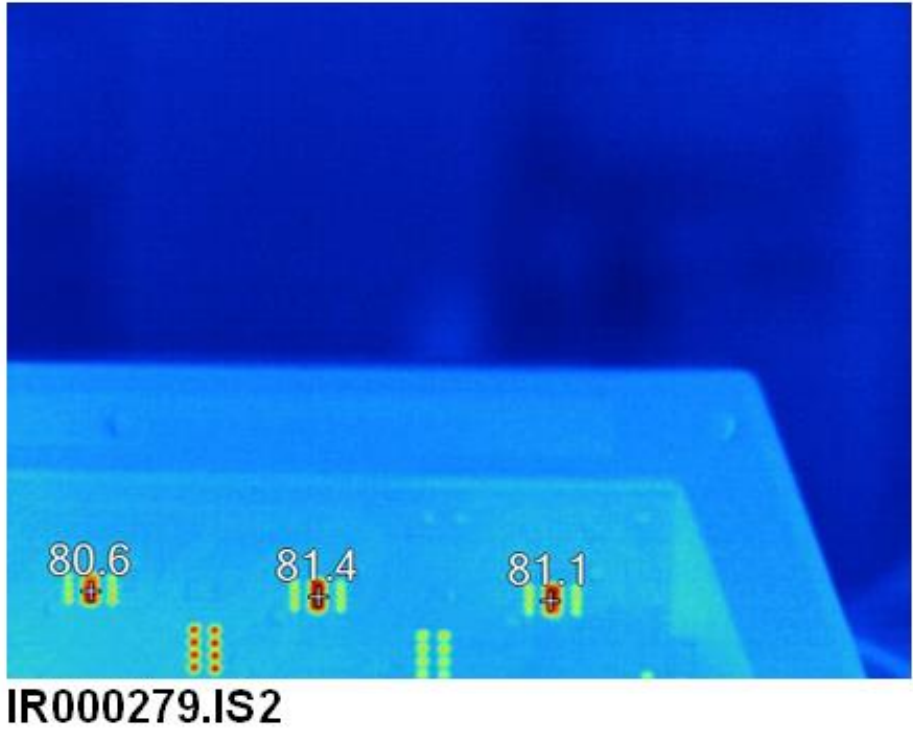
Şekil 12-6 Uzun hüzme modu çalışma koşulu için termal kamera ile ölçülen sıcaklık değerleri
