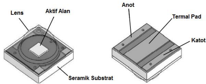
Şekil 6-5 Led katmanlarının ve termal yollarının şematik görünümü [8]
