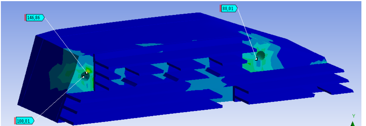
Şekil 8-2 Bağlantı arayüzündeki gerilim değerlerinin kontrolleri
