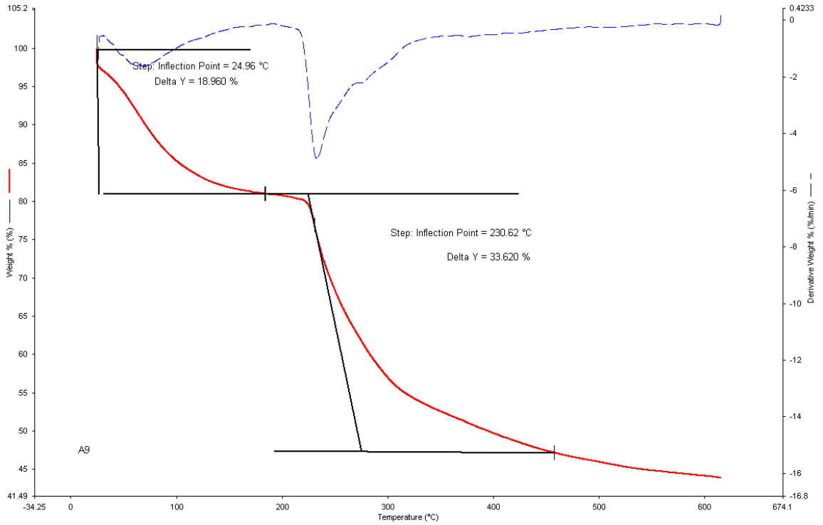
Şekil 6. 19 Aljinat – Kitosan Hibrit Küre (1:2) TGA analizi
