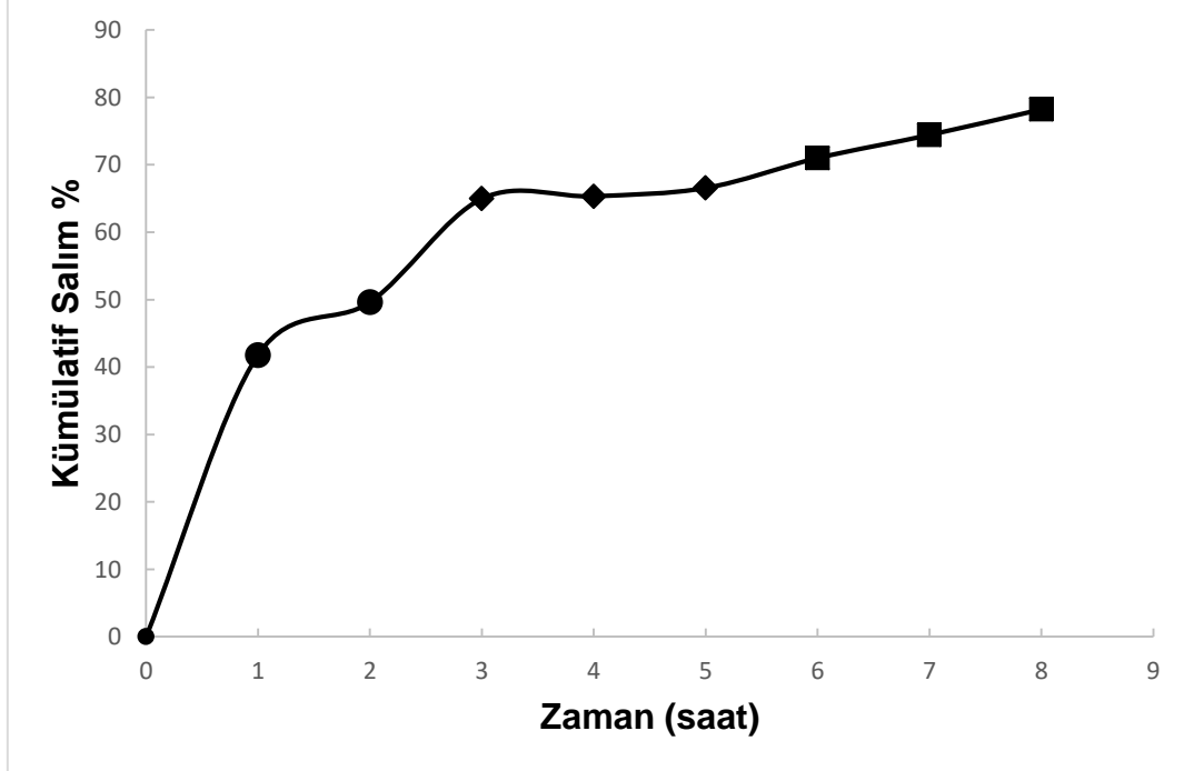
Şekil 6. 45 35 mg RSV yüklü 1:2 Oranındaki Aljinat – Kitosan hibrit kürelerin farklı tamponlardaki zamana karşı resveratrol salım profili
