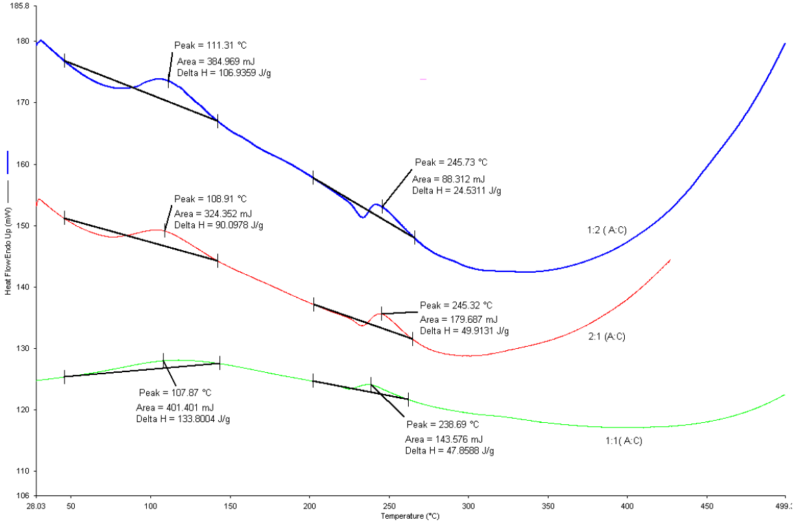
Şekil 6. 23 Aljinat – Kitosan Hibrit Kürelerin farklı kütle oranlarının DSC Analizleri, Yukarıdan aşağıya; (1:2), (2:1) ve (1:1)
