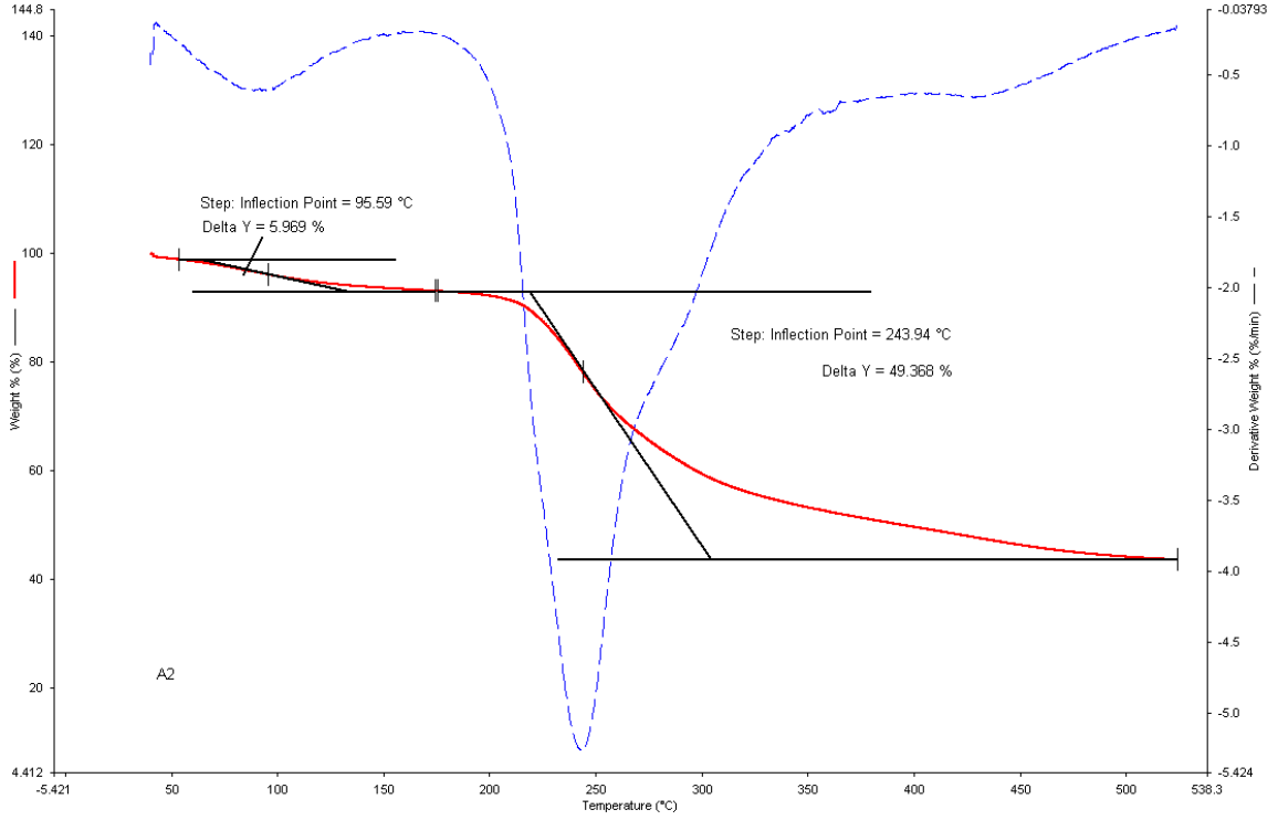
Şekil 6. 18 Aljinat – Kitosan Hibrit Küre (1:1) TGA analizi
