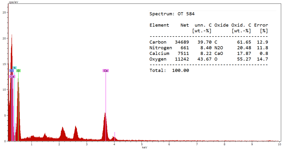
Şekil 6. 8 Yukarıdan aşağıya; Ca – Aljinat kürelerin EDS analizi ve Aljinat – Kitosan hibrit kürelerin EDS analizi
