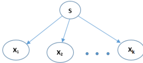
Şekil 2. Bağımsız Değişkenlerin ( x_1, x_2, \dots, x_k ), S Sınıflandırma Değişkenine Göre Koşullu Bağımsızlığını Gösteren Naive Bayes Modelinin Bayes Ağı Gösterimi
