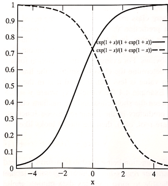
Şekil 9. Örnek Lojistik Eğri (Dunham, 2003, s. 86)
