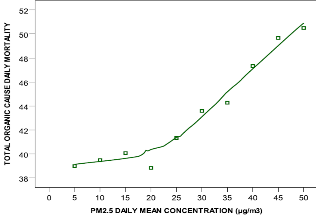
Şekil 2.8. PM 2.5 Konsantrasyonu Ve Toplam Doğal Ölümler Arasındaki Scatter-Plot Diyagramı [48]
