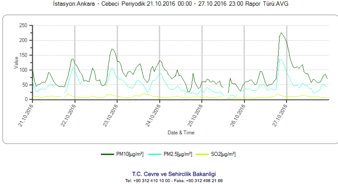
Şekil 5.19. 21-27 Ekim 2016 Ankara/Cebeci Hava Kalite Diyagramı
