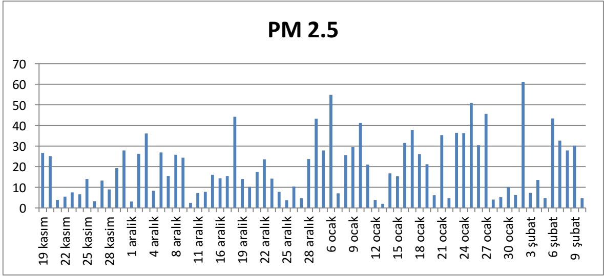
Şekil 4.2. PM 2.5 Konsantrasyonu Deney Döneminde Günlere Göre Dağılımı
