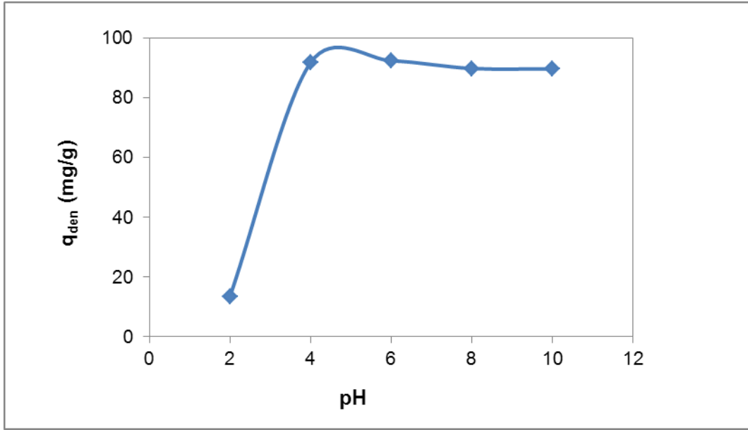
Şekil 5.47. MB'nun kurutulmuş şeker pancarı küspesine biyosorpsiyonunda, başlangıç pH'ının dengede birim biyosorbent kütlesi başına adsorplanan MB miktarına etkisi ( C_o=100 mg/l, T=25^\circ\text{C} , X_o=1 g/l, Karıştırma Hızı=100 rpm).
