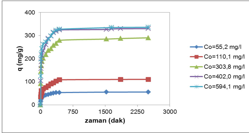
Şekil 5.30. pH 8.0'de RBB'nin 20 g/l CTAB ile yüzey modifikasyonu uygulanmış şeker pancarı küspesine biyosorpsiyonunda, farklı başlangıç RBB derişimlerinde elde edilen birim biyosorbent kütlesi başına adsorplanan RBB miktarının zamanla deęişim eğrileri (T=25°C, X 0 =1 g/l, tanecik boyut aralığı=500-707 µm, Karıştırma Hızı=100 rpm)
