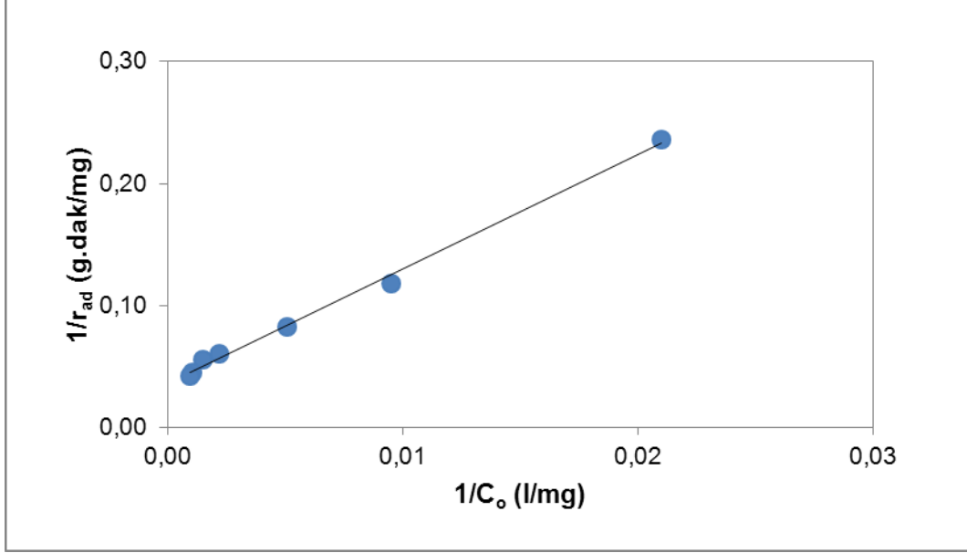
Şekil 5.17. pH 8.0'de RBB'nin 20 g/l CTAB ile modifikasyon uygulanmış R. arrhizus 'a biyosorpsiyonunda elde edilen 1/r_{ad} 'a karşı 1/C_o grafiği (T=25°C, X o =1 g/l, Karıştırma Hızı=100 rpm)
