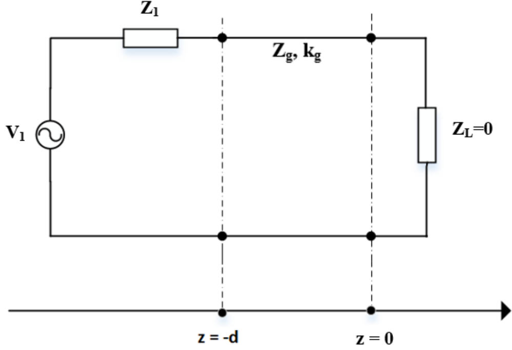
Şekil 2.6 Şekil 3.4'te bulunan iletim hattı modelinin sadeleştirilmiş hali
