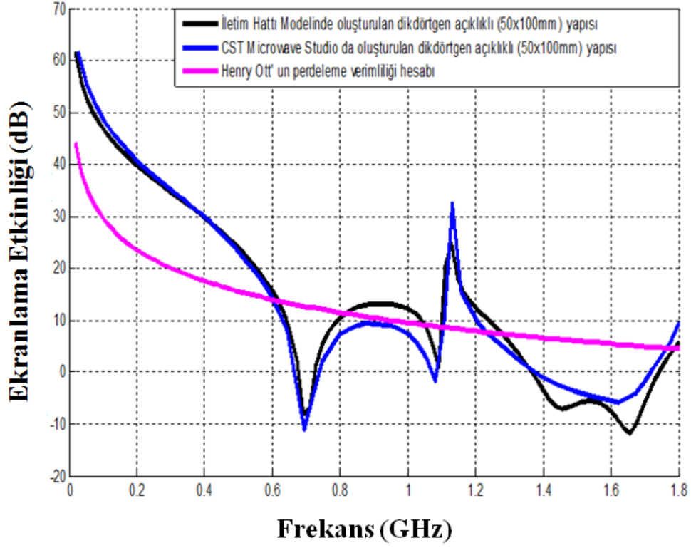
Şekil 3.6 Aynı özelliklerdeki ekranlama yapısı üzerine yerleştirilen dikdörtgen açıklıklı (50x100mm) sahip koruma yapılarının farklı yöntemler kullanılarak yapılan ekranlama verimliliği hesaplamaları
