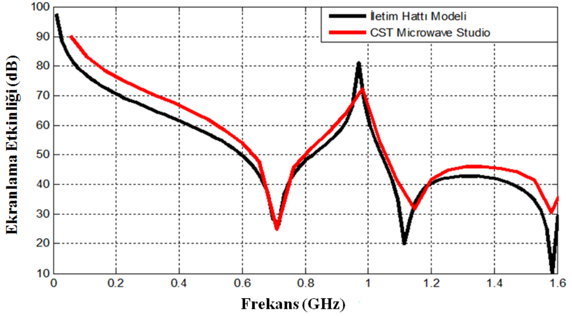
Şekil 3.28 Üzerinde dört tane 15x15 mm boyutlarında aralarında 10 mm mesafe bulunan kare açıklıklı ekranlama yapısı için Q(a/2, b/2, (-d/2)+30 \text{ mm}) noktasında ekranlama verimliliği hesaplaması
