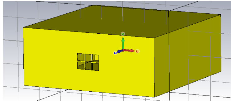
Şekil 3.29 Üzerinde altı tane 15x15 mm boyutlarında kare açıklık bulunan dikdörtgen prizma şeklindeki ekranlama yapısı
