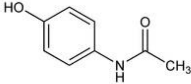
Şekil 2.1. N-(4-Hidroksifenil) asetamid yapısı.
