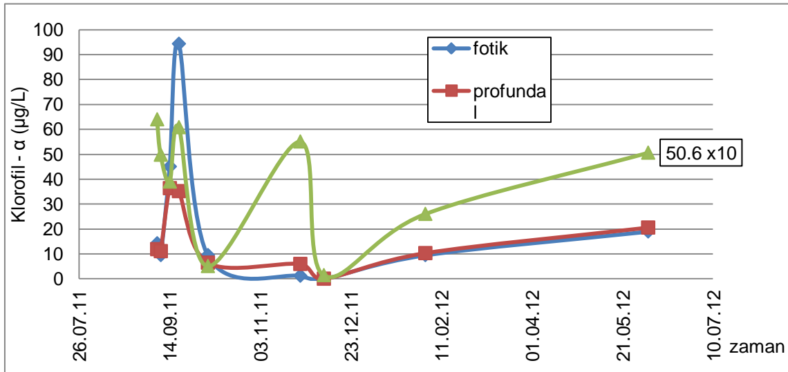
Şekil 5.36. Fotik, profundal ve bentik zonlarda klorofil-a konsantrasyonun zamanla değişimi.
