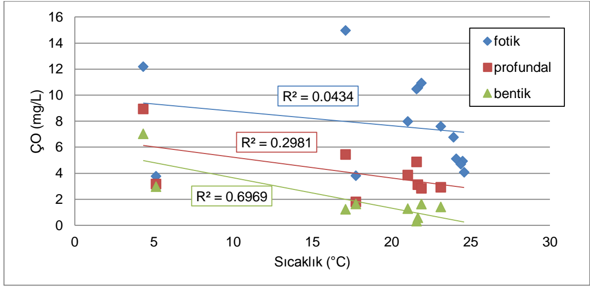
Şekil 5.28. Fotik, profundal ve bentik zonalarda ÇO-sıcaklık dağılım grafiği.
