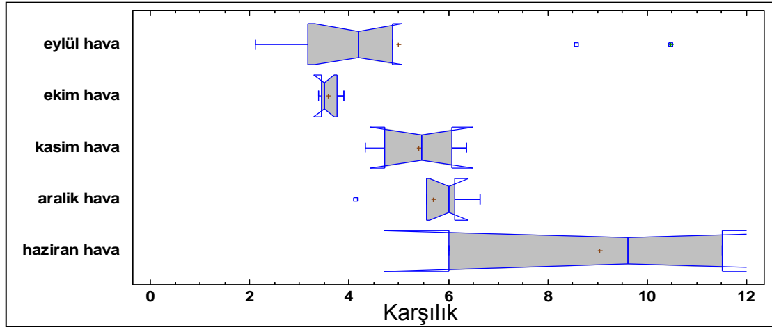
Şekil 5.116. Aylık hava fazında N_2O verilerinin ANOVA grafiği
