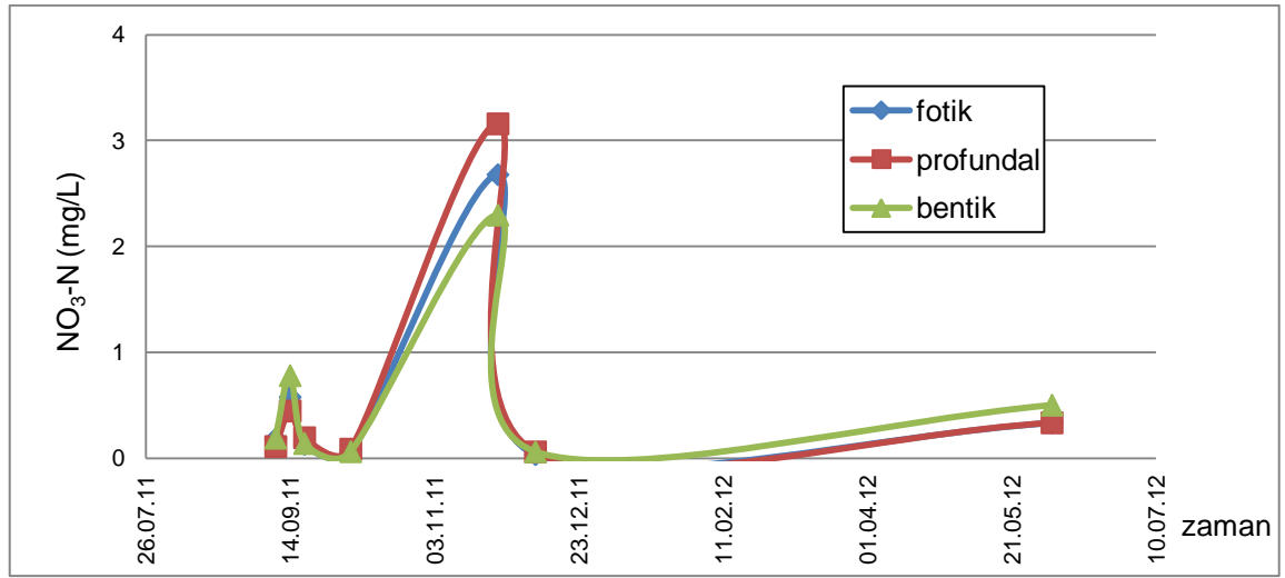
Şekil 5.42. Fotik, profundal ve bentik zonalarda \text{NO}_3\text{-N} konsantrasyonunun zamanla değişimi
