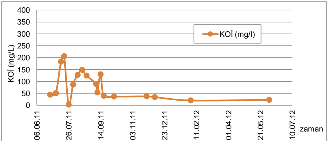
Şekil 5.41. Toplam KOİ konsantrasyonunun zamanla değişimi
