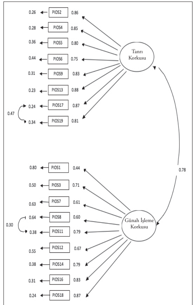
ŞEKİL 1. Penn Dinsel Obsesyonlar Envanteri'nin (PDOE) İki Faktörlü Yapısına İlişkin Modelin Standardize Değerleri.
