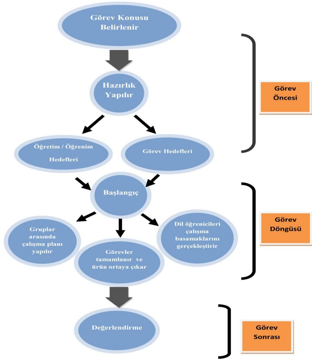
Şekil 2: Görev Şeması
